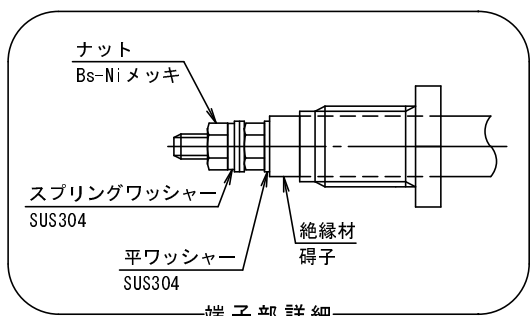
端子部詳細
