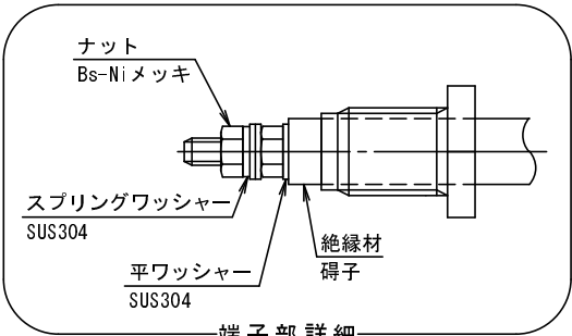
端子部詳細
